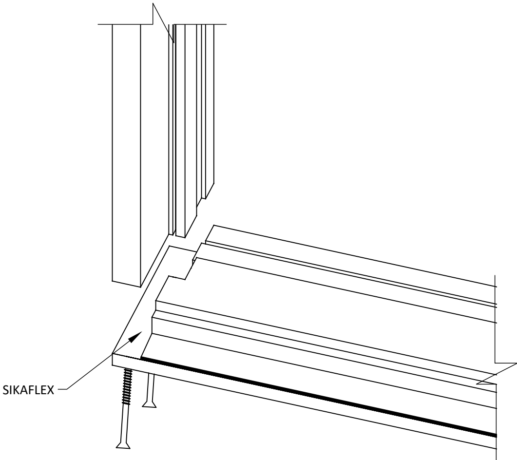
JAMB ASSEMBLY
